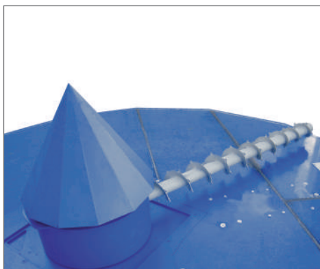
SBANCATORE A FRESA EXTRACTEUR A FRAISE WORM CONVEYOR FRÄSEVORRICHTUNG DESBANCADOR CON FRESA
