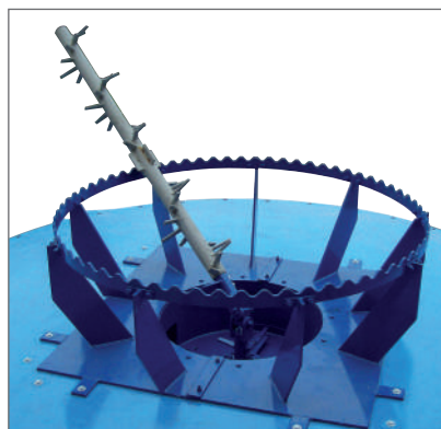
SBANCATORE ORBITALE EXTRACTEUR AVEC UN ARBRE INCLINÉ SLANTED ARM CONVEYOR SCHRÄGRÜHRVORRICHTUNG DESBANCADOR CON ÁRBOL INCLINADO
